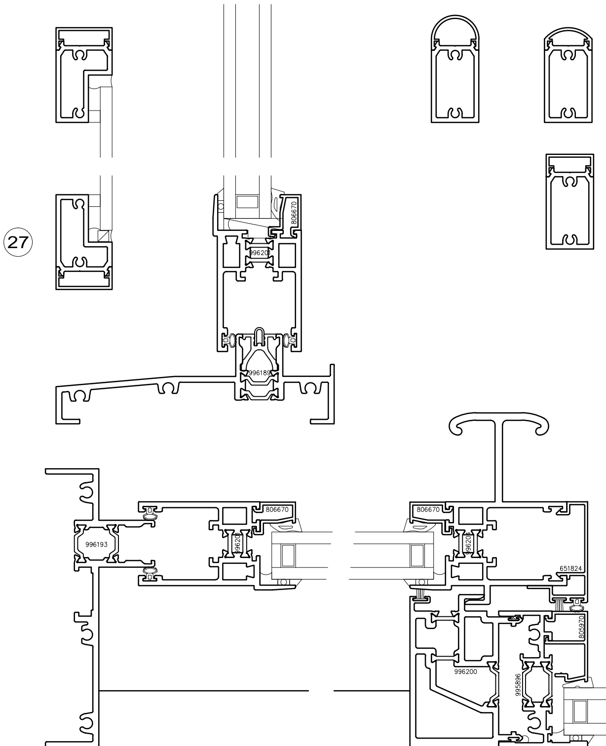
Juliet Balcony
