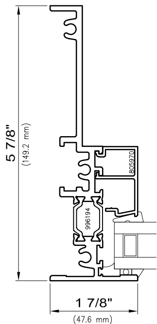
8 Fixed Jamb Inside Slide
